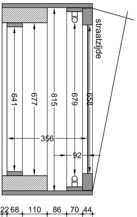
vooraanzicht
